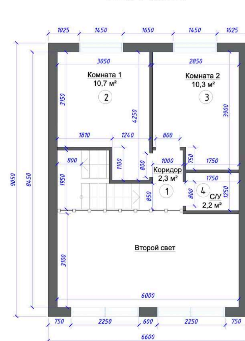
План 2 этажа
