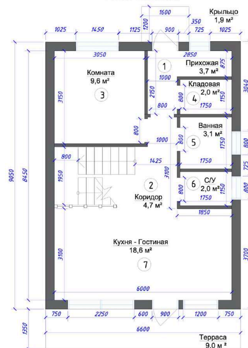
План 1 этажа
