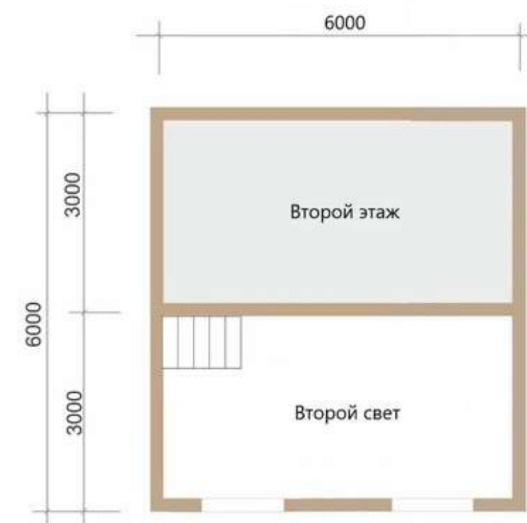
План 2 этажа
